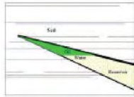
Pinchout
