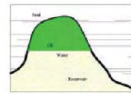
Reef
